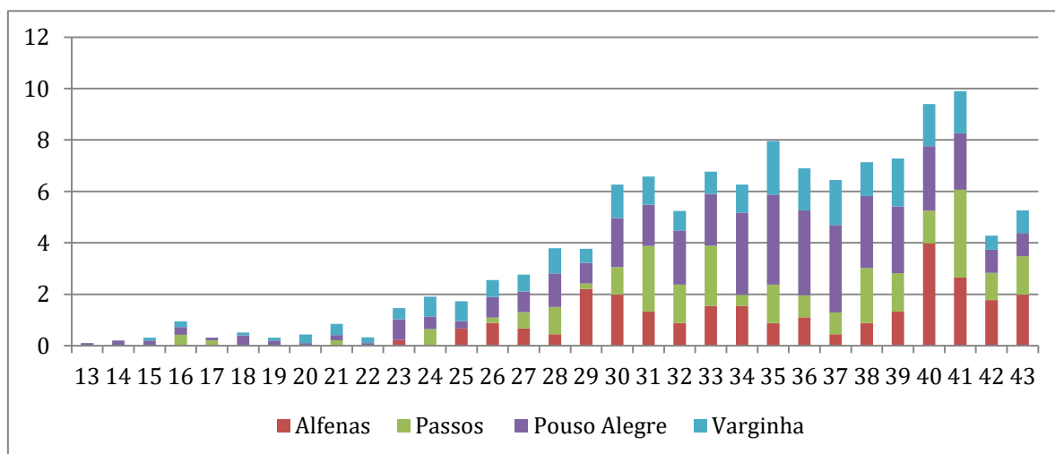
Gráfico 07- Coeficientes de mortalidade por COVID por SRS de residência e semana epidemiológica de ocorrência (22/03 a 24/10). Macrorregião Sul de Saúde, 2020.
