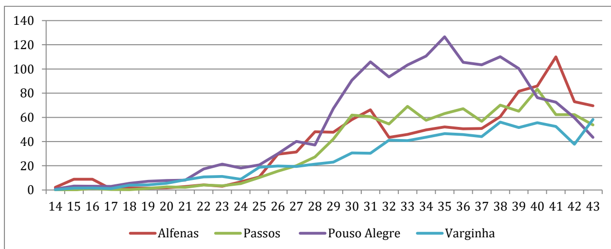
Gráfico 06- Coeficientes de incidência por COVID-19 por SRS de residência e semana epidemiológica (12/04 a 24/10), Macrorregião Sul de Saúde - MG.
